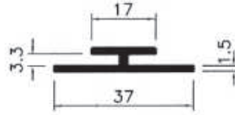
3614 0,236 kg/m
