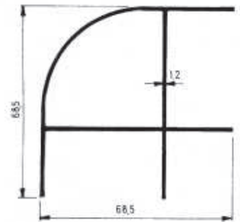
3622 0,796 kg/m
