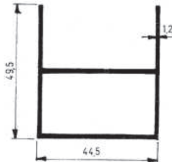
3623 0,593 kg/m
