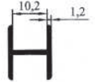
3619 0,135 kg/m
