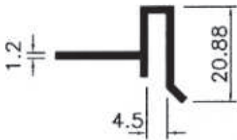
3616 0,194 kg/m
