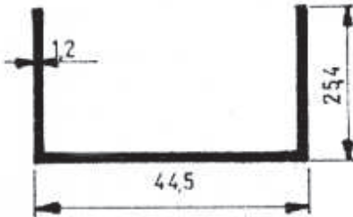
3620 0,300 kg/m
