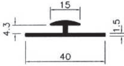
3613 0,251 kg/m
