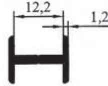
3618 0,140 kg/m
