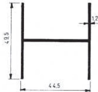
3621 0,490 kg/m
