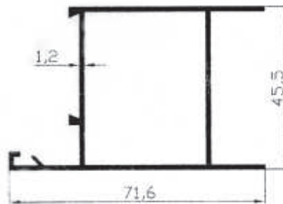
3624 0,708 kg/m
