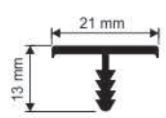
2610 0,158 kg/m
