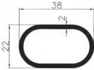
2714 0,513 kg/m
