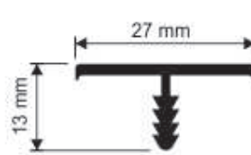
2609 0,183 kg/m
