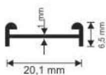
2623 0,096 kg/m
