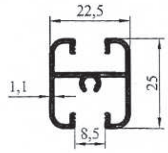
4023 0,328 gr/m
