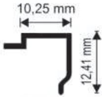
2664 0,69 kg/m
