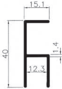
2724 0,324 kg/m
