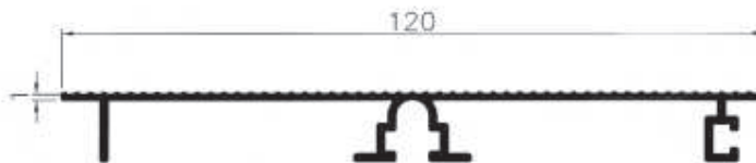
2722 0,597 kg/m
