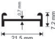
2622 0,083 kg/m
